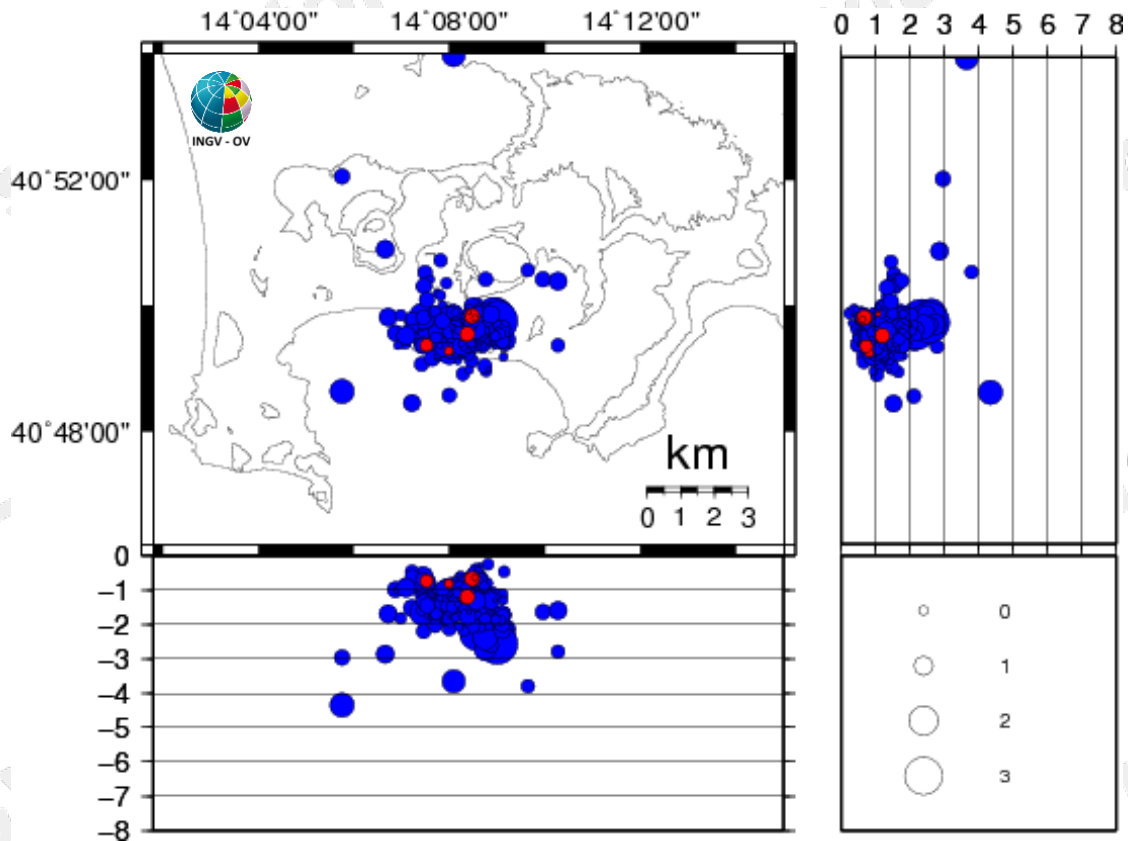
Figura 3.1 - Ipocentri dei terremoti localizzati ai Campi Flegrei negli ultimi 12 mesi (in totale 572). In rosso gli eventi localizzati nell'ultima settimana (in totale 6).
