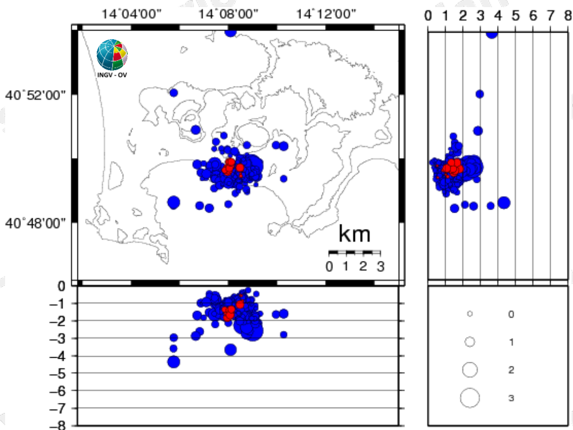
Figura 3.1 - Ipocentri dei terremoti localizzati ai Campi Flegrei negli ultimi 12 mesi (in totale 594). In rosso gli eventi localizzati nell'ultima settimana (in totale 16).
