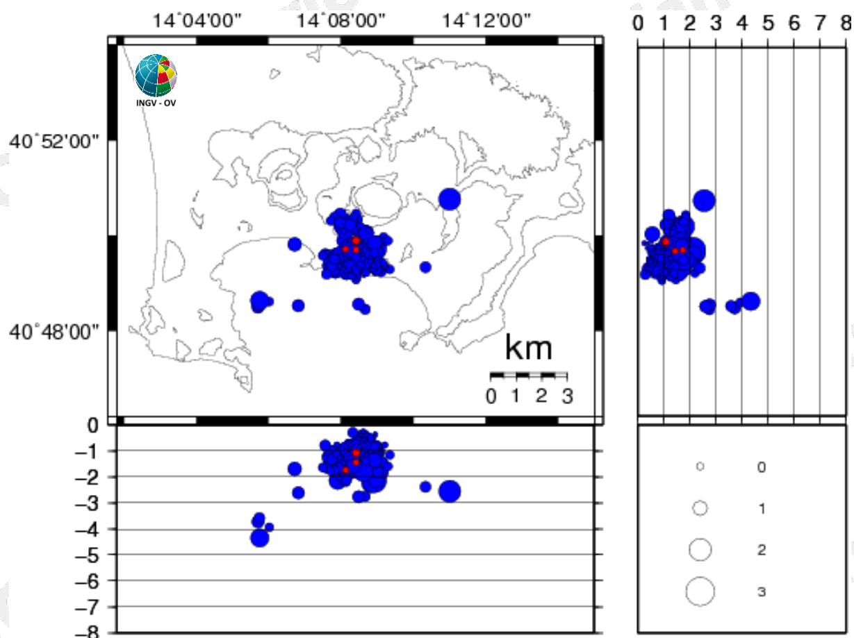
Figura 3.1 - Ipocentri dei terremoti localizzati ai Campi Flegrei negli ultimi 12 mesi (in totale 427). In rosso gli eventi localizzati nell'ultima settimana (in totale 3).
