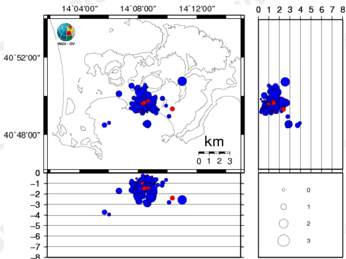
Figura 3.1 - Ipocentri dei terremoti localizzati ai Campi Flegrei negli ultimi 12 mesi (in totale 344). In rosso gli eventi localizzati nell'ultima settimana (in totale 6).
