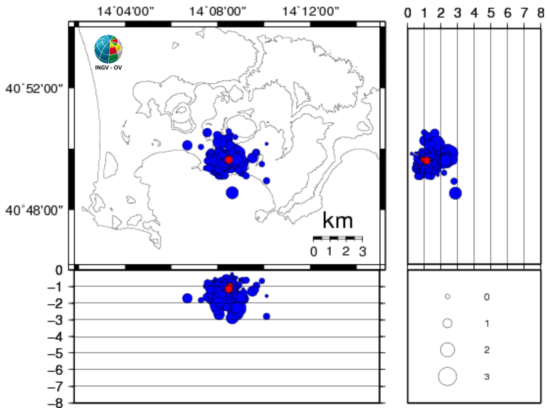
Figura 3.1 - Ipocentri dei terremoti localizzati ai Campi Flegrei negli ultimi 12 mesi (in totale 302). In rosso gli eventi localizzati nell'ultima settimana (in totale 2).
