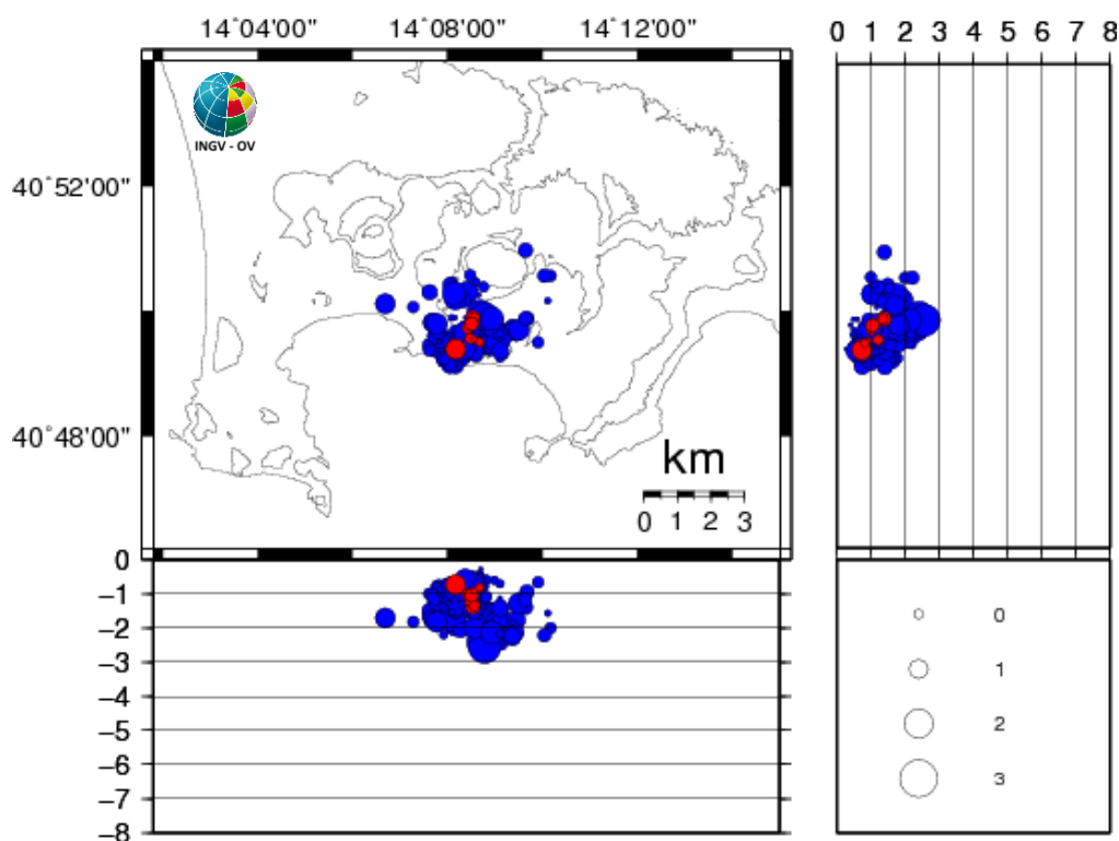
Figura 1.1 - Ipocentri dei terremoti localizzati ai Campi Flegrei negli ultimi 12 mesi (in totale 235). In rosso gli eventi localizzati nell'ultima settimana (in totale 8).
