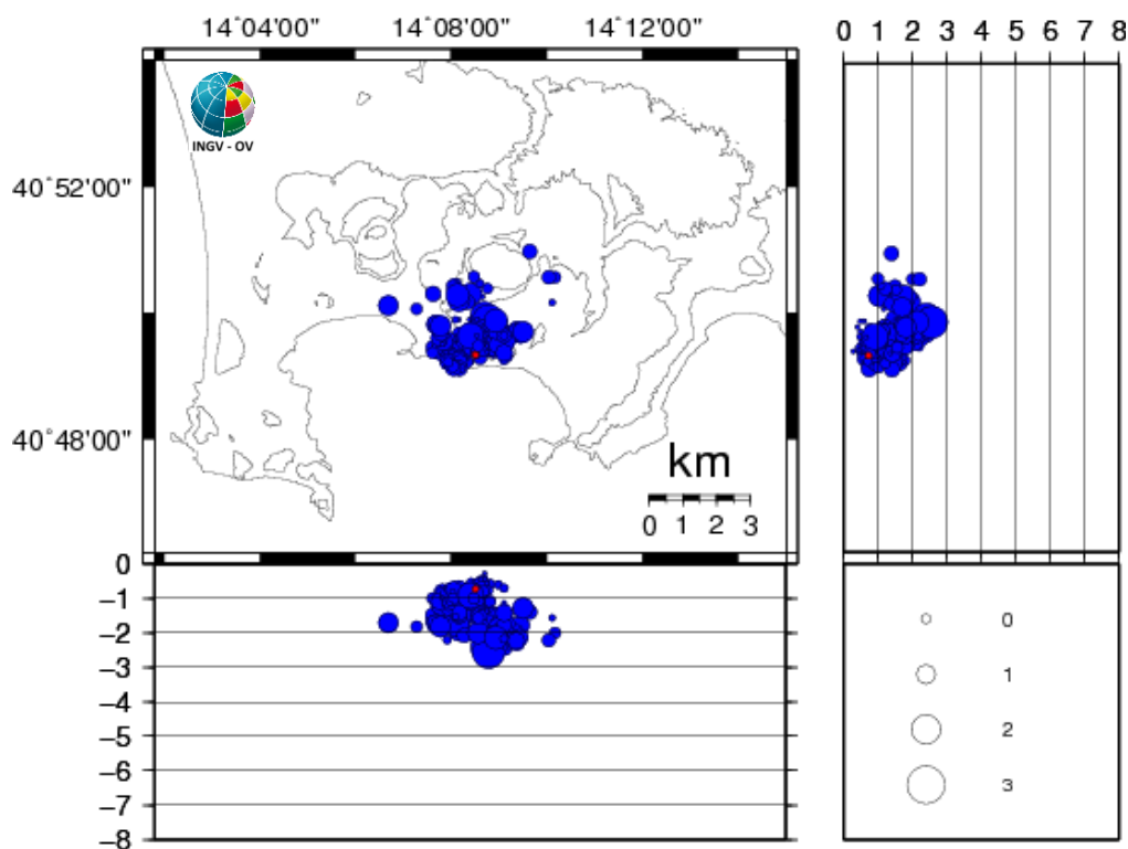
Figura 1.1 - Ipocentri dei terremoti localizzati ai Campi Flegrei negli ultimi 12 mesi (in totale 216). In rosso gli eventi localizzati nell'ultima settimana (in totale 1).
