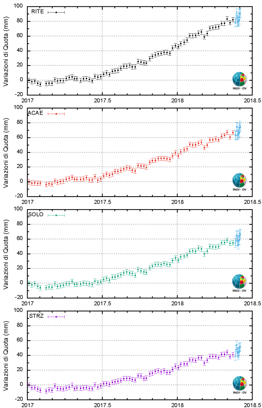
Figura 2.2 - Serie temporali delle variazioni in quota delle stazioni di RITE (Pozzuoli – Rione Terra), ACAE (Accademia Aeronautica), SOLO (Solfatarara) e STRZ (Pozzuoli - Cimitero) dal 01 gennaio 2017 al 04 giugno 2018.
