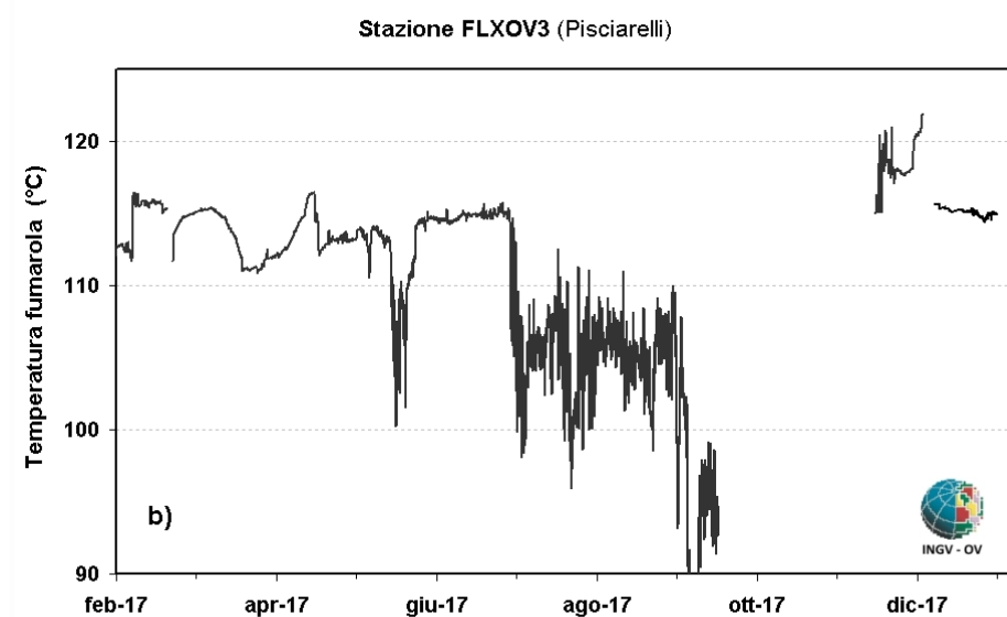
Figura 3.1 - (a) Valori del flusso di CO 2 dal suolo (medie giornaliere); (b) dettaglio della temperatura della fumarola dal mese di febbraio.
