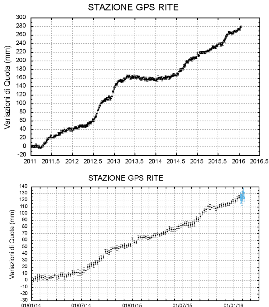
Figura 2 - Serie temporale delle variazioni in quota della stazione di RITE (Pozzuoli) dal 01 gennaio 2011 al 23 gennaio 2016 (in alto) e dal 01 gennaio 2014 al 08 febbraio 2016 (in basso).
