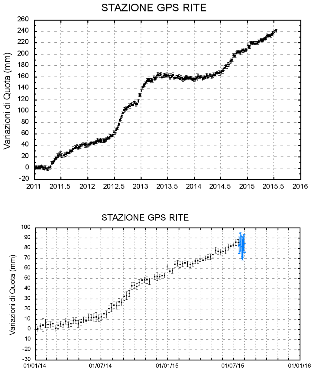
Figura 2 - Serie temporale delle variazioni in quota della stazione di RITE (Pozzuoli) dal 01 gennaio 2011 al 18 luglio 2015 (in alto) e dal 01 gennaio 2014 al 02 agosto 2015 (in basso).
