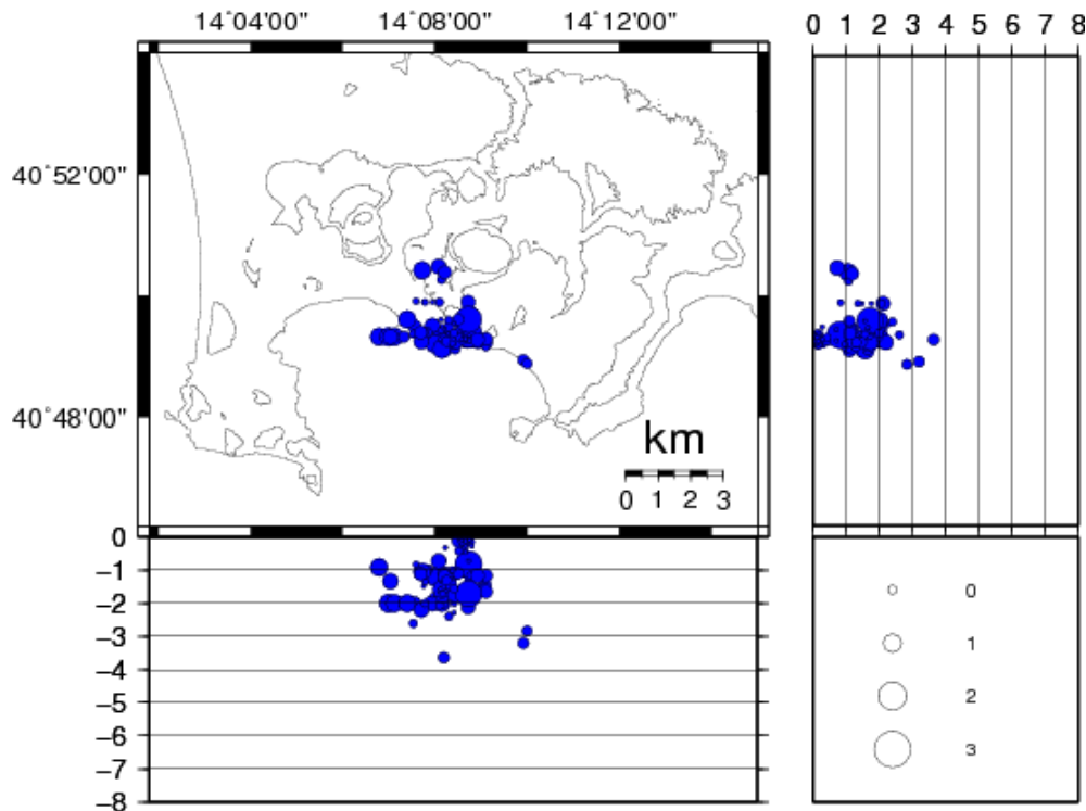
Figura 1 - Ipocentri dei terremoti localizzati ai Campi Flegrei negli ultimi 12 mesi (in totale 113).
