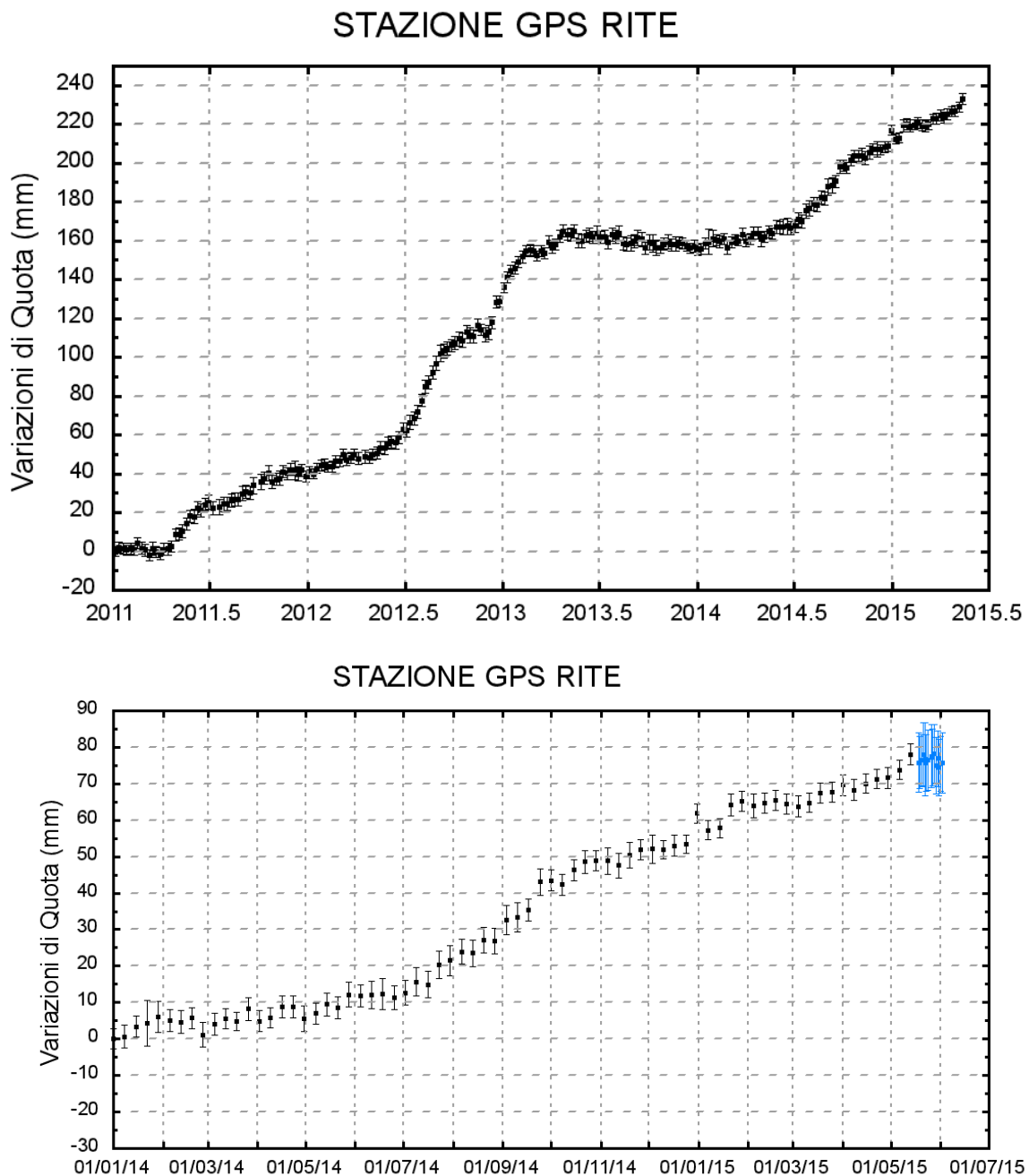
Figura 2 - Serie temporale delle variazioni in quota della stazione di RITE (Pozzuoli) dal 01 gennaio 2011 al 09 maggio 2015 (in alto) e dal 01 gennaio 2014 al 02 giugno 2015 (in basso).
