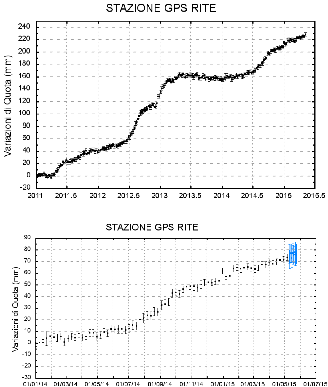
Figura 2 - Serie temporale delle variazioni in quota della stazione di RITE (Pozzuoli) dal 01 gennaio 2011 al 09 maggio 2015 (in alto) e dal 01 gennaio 2014 al 25 maggio 2015 (in basso).
