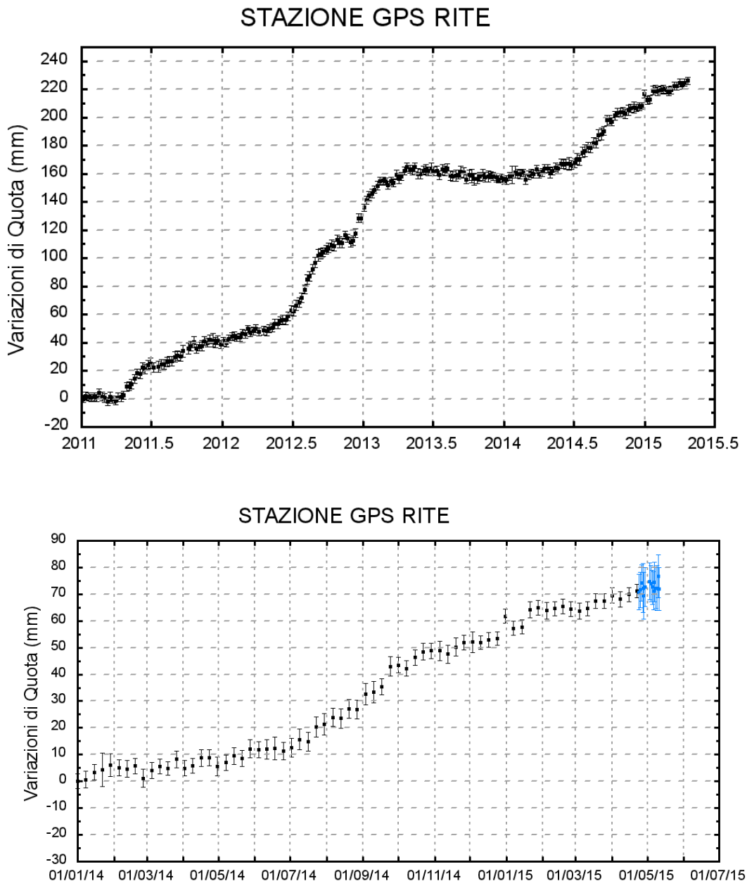
Figura 2 - Serie temporale delle variazioni in quota della stazione di RITE (Pozzuoli) dal 01 gennaio 2011 al 25 aprile 2015 (in alto) e dal 01 gennaio 2014 al 11 maggio 2015 (in basso).
