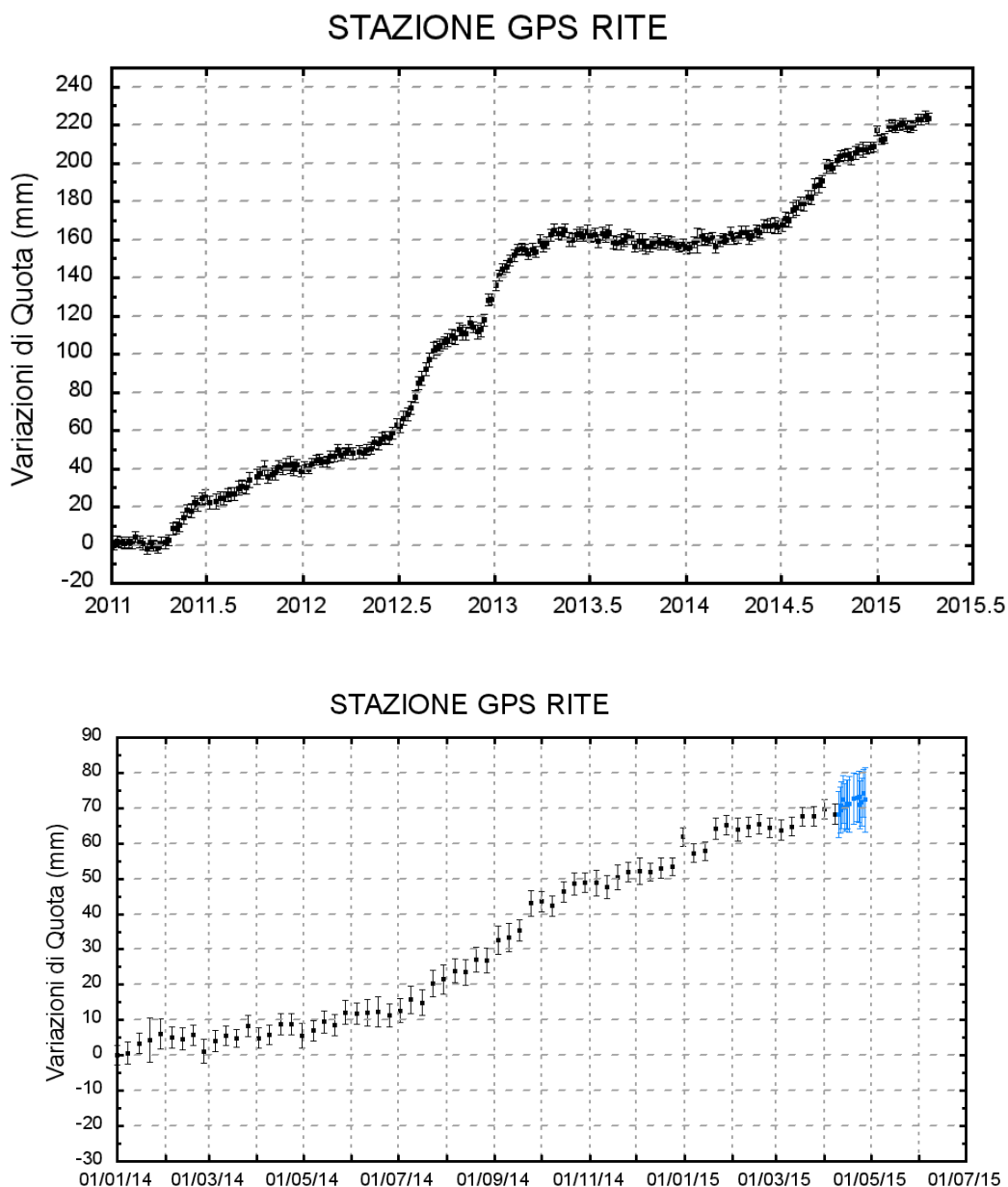
Figura 2 - Serie temporale delle variazioni in quota della stazione di RITE (Pozzuoli) dal 01 gennaio 2011 al 11 aprile 2015 (in alto) e dal 01 gennaio 2014 al 27 aprile 2015 (in basso).
