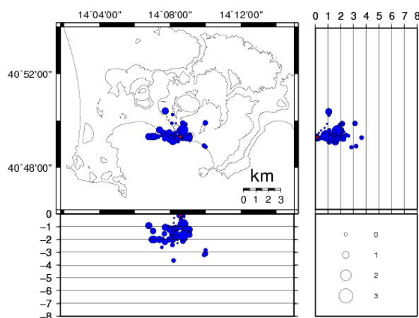
Figura 1 - Ipocentri dei terremoti localizzati ai Campi Flegrei negli ultimi 12 mesi (in totale 106). Quelli avvenuti nell'ultima settimana sono colorati in rosso (in totale 1).
