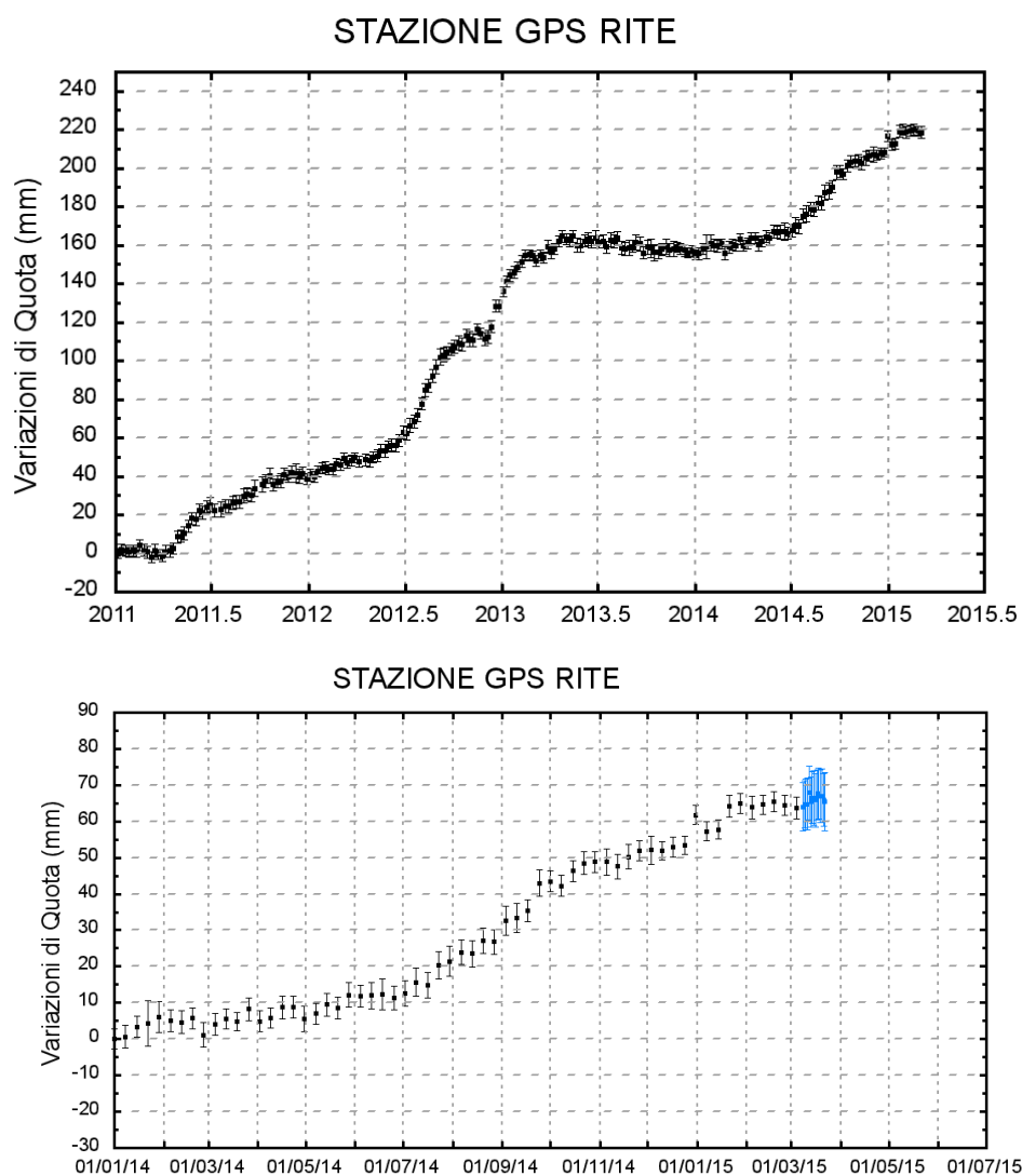
Figura 2 - Serie temporale delle variazioni in quota della stazione di RITE (Pozzuoli) dal 01 gennaio 2011 al 07 marzo 2015 (in alto) e dal 01 gennaio 2014 al 23 marzo 2015 (in basso).
