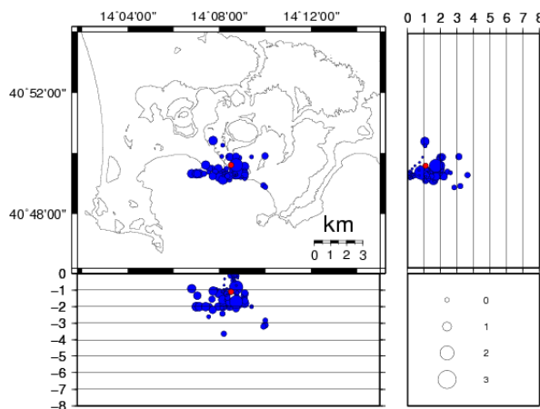
Figura 1 - Ipocentri dei terremoti localizzati ai Campi Flegrei negli ultimi 12 mesi (in totale 103). In rosso l'evento localizzato nell'ultima settimana.
