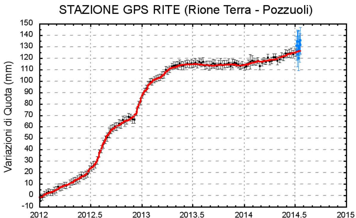
Figura 2 - Serie temporale delle variazioni in quota della stazione di RITE (Pozzuoli) dal 01 gennaio 2012 al 21 luglio 2014.
