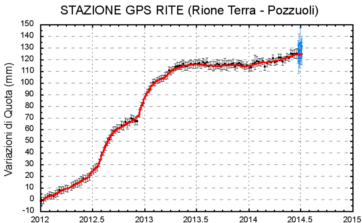
Figura 2 - Serie temporale delle variazioni in quota della stazione di RITE (Pozzuoli) dal 01 gennaio 2012 al 07 luglio 2014.
