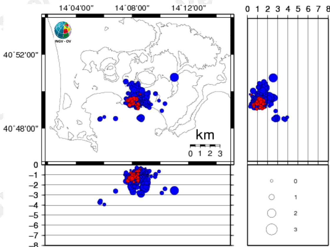
Figura 3.1 - Ipocentri dei terremoti localizzati ai Campi Flegrei negli ultimi 12 mesi (in totale 424). In rosso gli eventi localizzati nell'ultima settimana (in totale 28).
