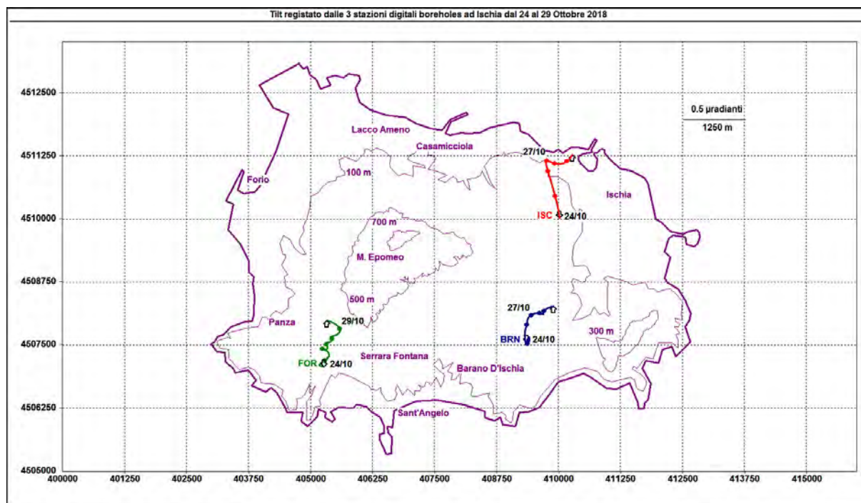
Figura 2.9 - Pattern tiltmetrico osservato dal 24 al 29 Ottobre. Il lato di ogni maglia del reticolo equivale a 0.5 \mu\text{radianti} o 1250 \text{ m} . I pallini in colore sovrapposti sui vettori tilt indicano l'inizio di ogni giorno.
