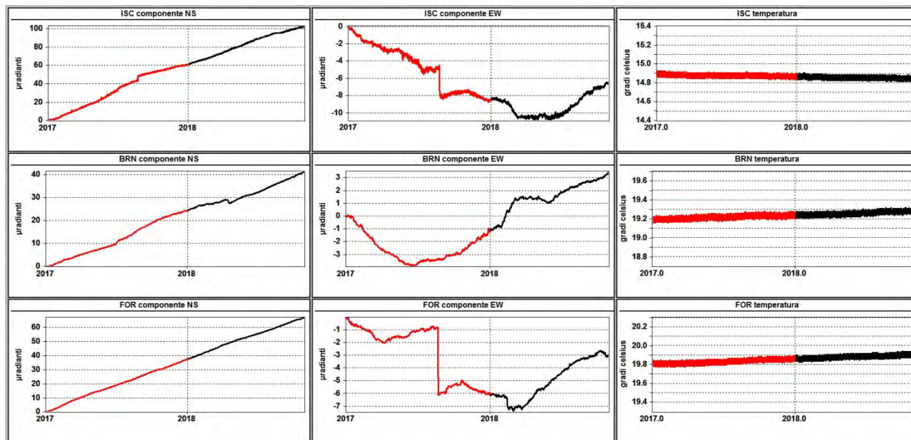
Figura 2.6 – Serie temporali dei segnali registrati a partire da gennaio 2017 dalle 3 stazioni “borehole” della Rete Tiltmetrica di Ischia, con sensori ubicati a 25 m di profondità, ordinate dal basso verso l’alto secondo la latitudine. Le prime 2 colonne riportano le componenti NS ed EW in \mu radianti i cui valori di tilt crescenti nel tempo indicano rispettivamente la variazione di inclinazione del suolo a N e ad E, mentre la terza colonna riporta la temperatura in ^{\circ} C registrata da ogni sensore. In rosso sono riportati i segnali relativi al 2017 mentre in nero sono rappresentati quelli registrati nel 2018.
