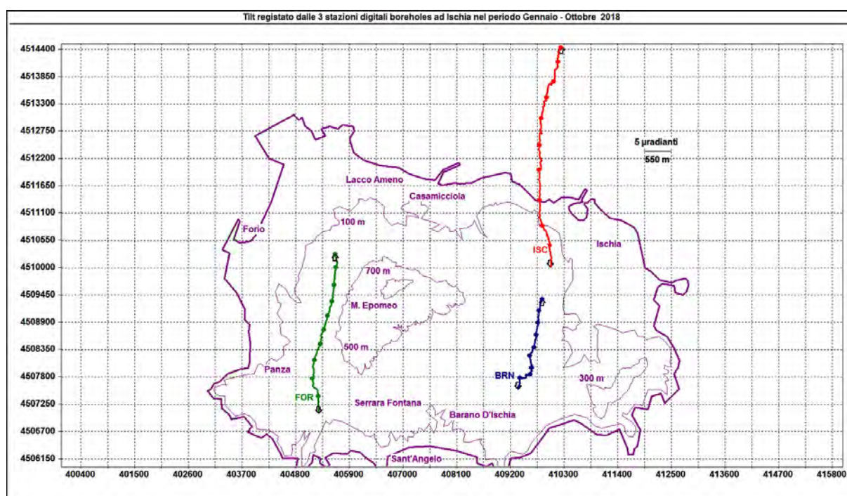
Figura 2.5 – Pattern tiltmetrico osservato ad Ischia nel periodo gennaio-ottobre 2018. Il lato di ogni maglia del reticolo equivale a 5 \mu radianti o 550 m. I pallini sovrapposti sui vettori tilt indicano l'inizio di ogni mese.
