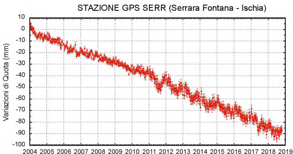
Figura 2.2 - Serie temporale delle variazioni settimanali in quota della stazione di SERR (Ischia) dal 2004 a ottobre 2018.
