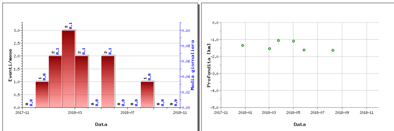
Figura 1.3 – (A sinistra) Numero di eventi registrati ad Ischia nel corso degli ultimi 12 mesi (in totale 11). (A destra) Profondità ipocentrali degli eventi registrati ad Ischia nel corso degli ultimi 12 mesi.
