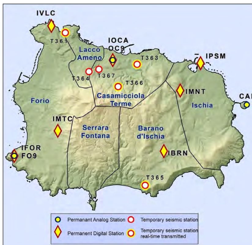
Figura 3.1 – Mappa della Rete Sismica Mobile installata ad Ischia ad integrazione della Rete Permanente.
