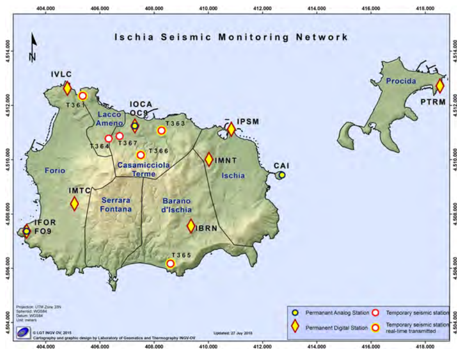
Figura 1.1 - Mappa della Rete Sismica di Ischia.
