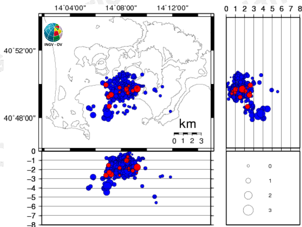
Figura 3.1 - Ipocentri dei terremoti localizzati ai Campi Flegrei negli ultimi 12 mesi (in totale 1152). In rosso gli eventi localizzati nell'ultima settimana (in totale 19).
