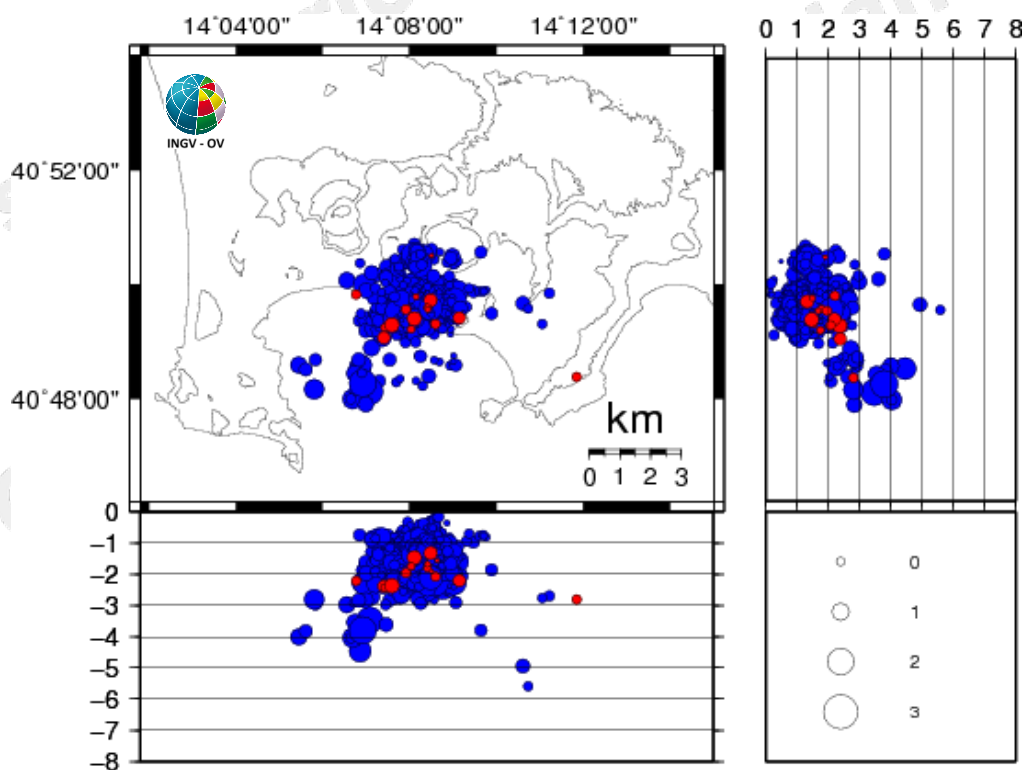
Figura 3.1 - Ipocentri dei terremoti localizzati ai Campi Flegrei negli ultimi 12 mesi (in totale 1175). In rosso gli eventi localizzati nell'ultima settimana (in totale 16).
