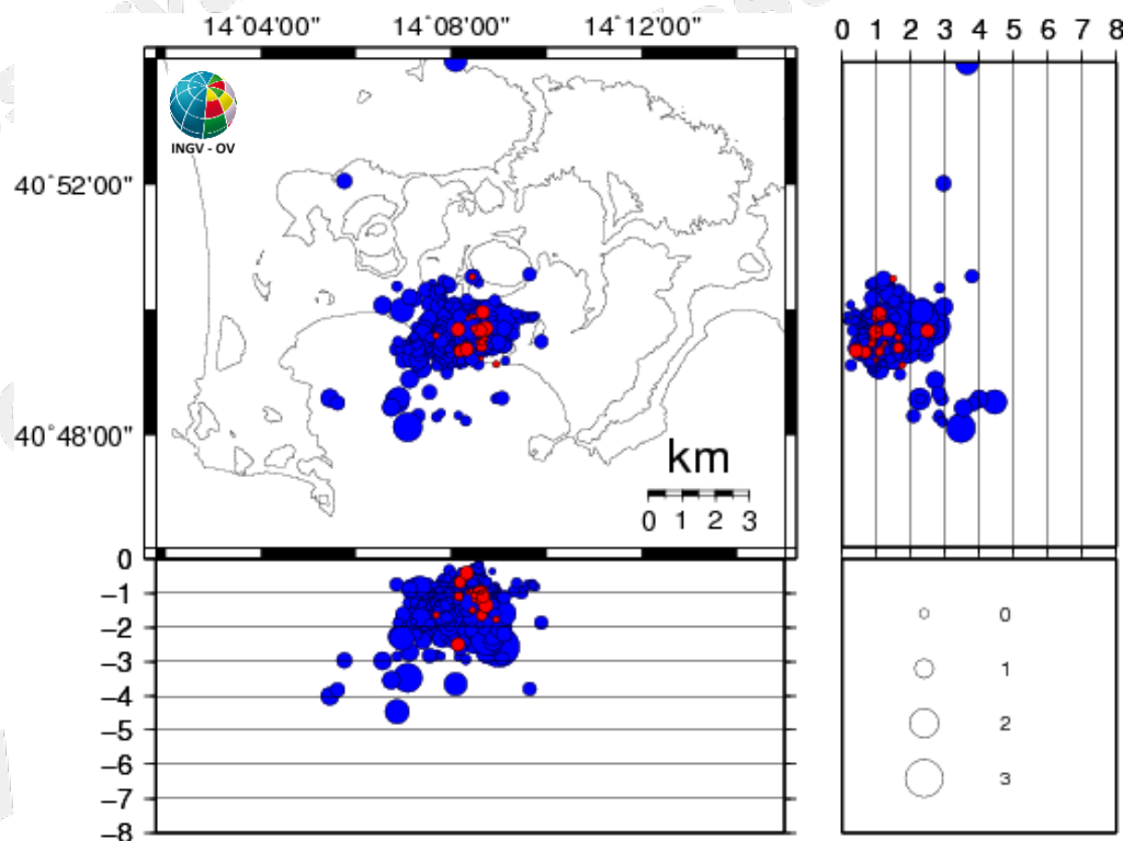
Figura 3.1 - Ipocentri dei terremoti localizzati ai Campi Flegrei negli ultimi 12 mesi (in totale 991). In rosso gli eventi localizzati nell'ultima settimana (in totale 34).
