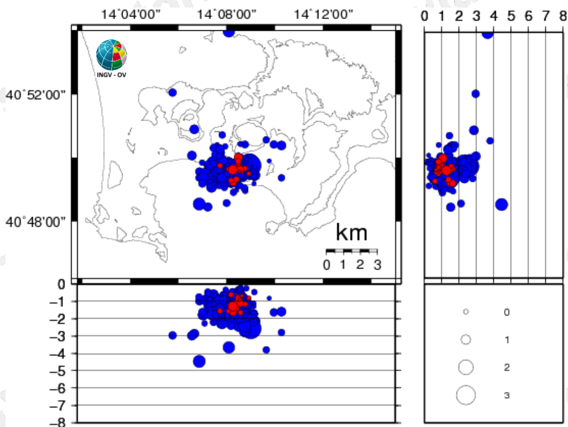
Figura 3.1 - Ipocentri dei terremoti localizzati ai Campi Flegrei negli ultimi 12 mesi (in totale 847). In rosso gli eventi localizzati nell'ultima settimana (in totale 28).
