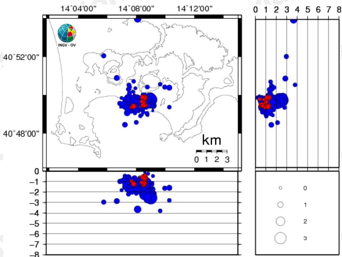
Figura 3.1 - Ipocentri dei terremoti localizzati ai Campi Flegrei negli ultimi 12 mesi (in totale 642). In rosso gli eventi localizzati nell'ultima settimana (in totale 22).
