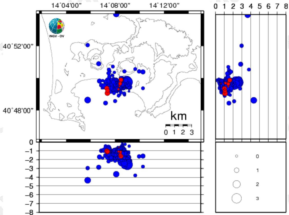
Figura 3.1 - Ipocentri dei terremoti localizzati ai Campi Flegrei negli ultimi 12 mesi (in totale 567). In rosso gli eventi localizzati nell'ultima settimana (in totale 10).
