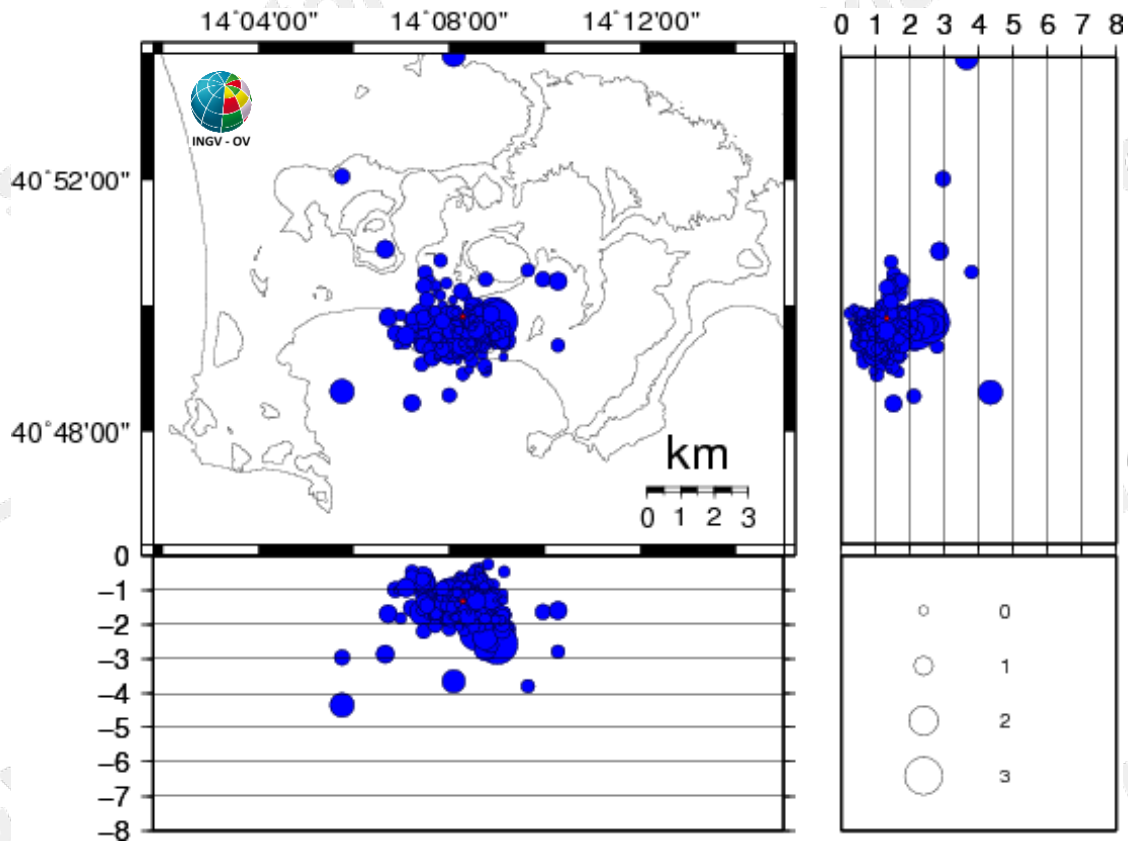
Figura 3.1 - Ipocentri dei terremoti localizzati ai Campi Flegrei negli ultimi 12 mesi (in totale 565). In rosso gli eventi localizzati nell'ultima settimana (in totale 1).
