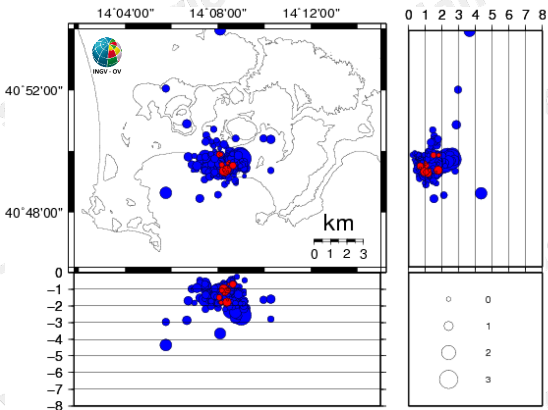
Figura 3.1 - Ipocentri dei terremoti localizzati ai Campi Flegrei negli ultimi 12 mesi (in totale 571). In rosso gli eventi localizzati nell'ultima settimana (in totale 13).
