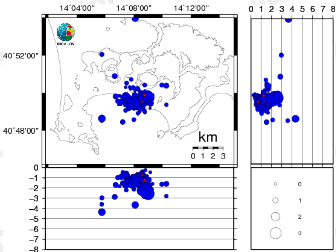
Figura 3.1 - Ipocentri dei terremoti localizzati ai Campi Flegrei negli ultimi 12 mesi (in totale 579). In rosso gli eventi localizzati nell'ultima settimana (in totale 3).
