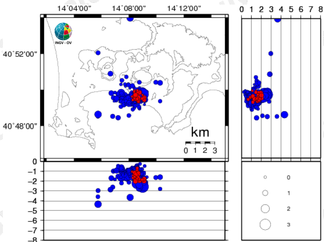
Figura 3.1 - Ipocentri dei terremoti localizzati ai Campi Flegrei negli ultimi 12 mesi (in totale 578). In rosso gli eventi localizzati nell'ultima settimana (in totale 36).
