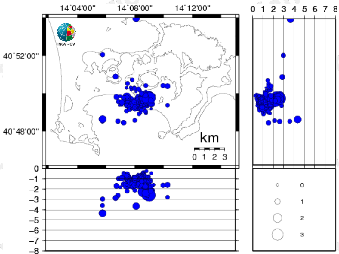
Figura 3.1 - Ipocentri dei terremoti localizzati ai Campi Flegrei negli ultimi 12 mesi (in totale 542).
