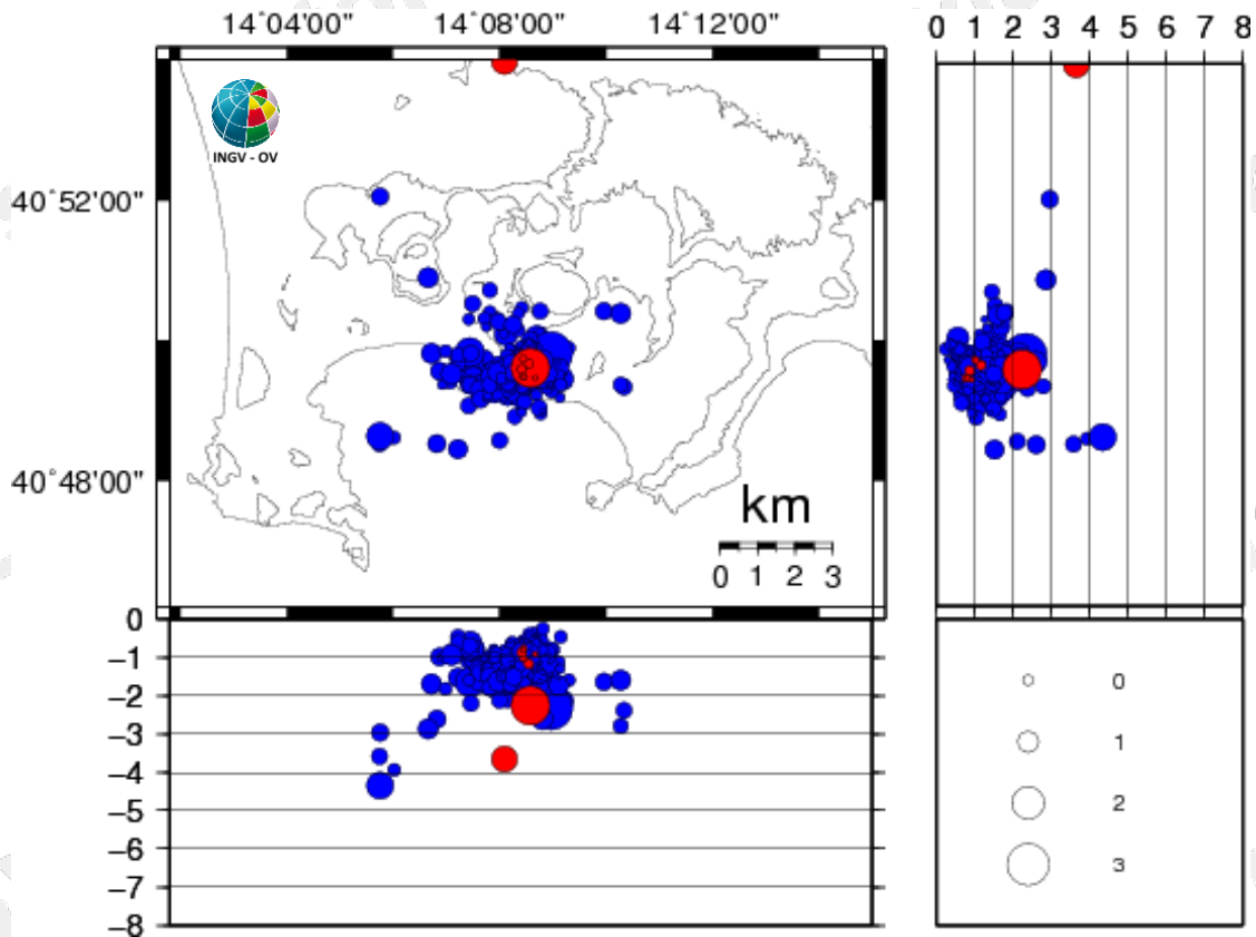
Figura 3.1 - Ipocentri dei terremoti localizzati ai Campi Flegrei negli ultimi 12 mesi (in totale 529). In rosso gli eventi localizzati nell'ultima settimana (in totale 8).
