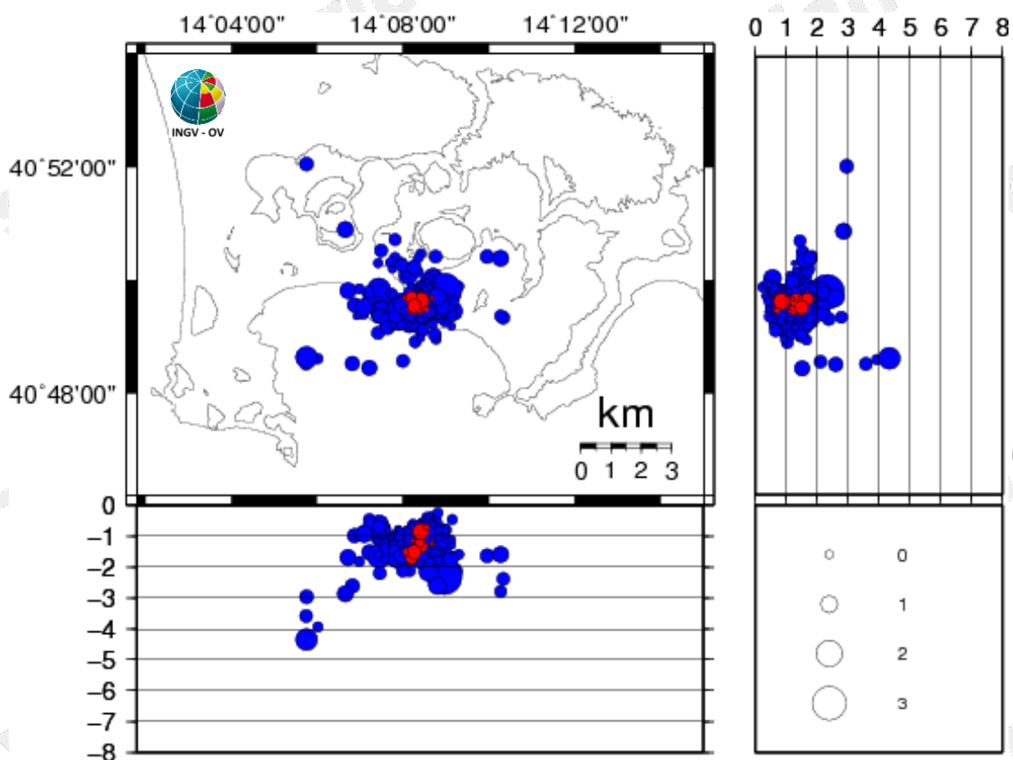
Figura 3.1 - Ipocentri dei terremoti localizzati ai Campi Flegrei negli ultimi 12 mesi (in totale 521). In rosso gli eventi localizzati nell'ultima settimana (in totale 11).
