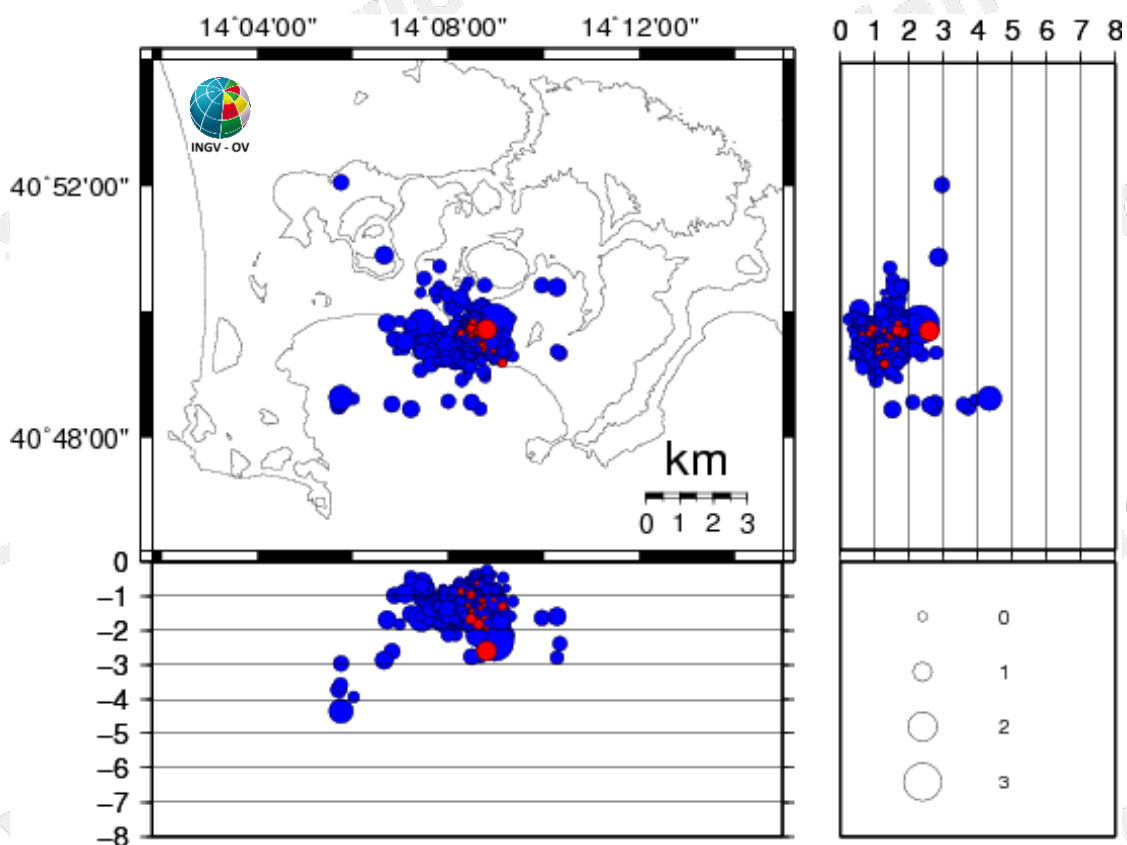
Figura 3.1 - Ipocentri dei terremoti localizzati ai Campi Flegrei negli ultimi 12 mesi (in totale 570). In rosso gli eventi localizzati nell'ultima settimana (in totale 20).
