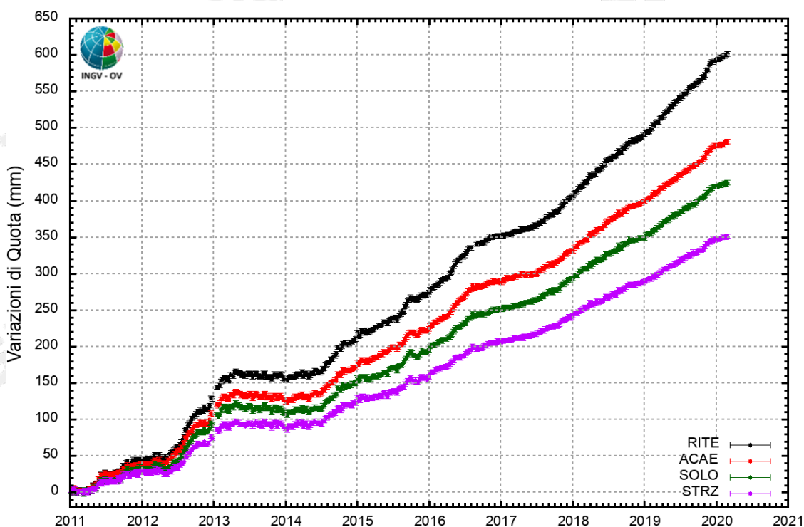
Figura 4.1 - Serie temporali delle variazioni in quota delle stazioni di RITE (Pozzuoli – Rione Terra), ACAE (Accademia Aeronautica), SOLO (Solfatarata) e STRZ (Pozzuoli - Cimitero) dal 01 gennaio 2011 al 29 febbraio 2020.
