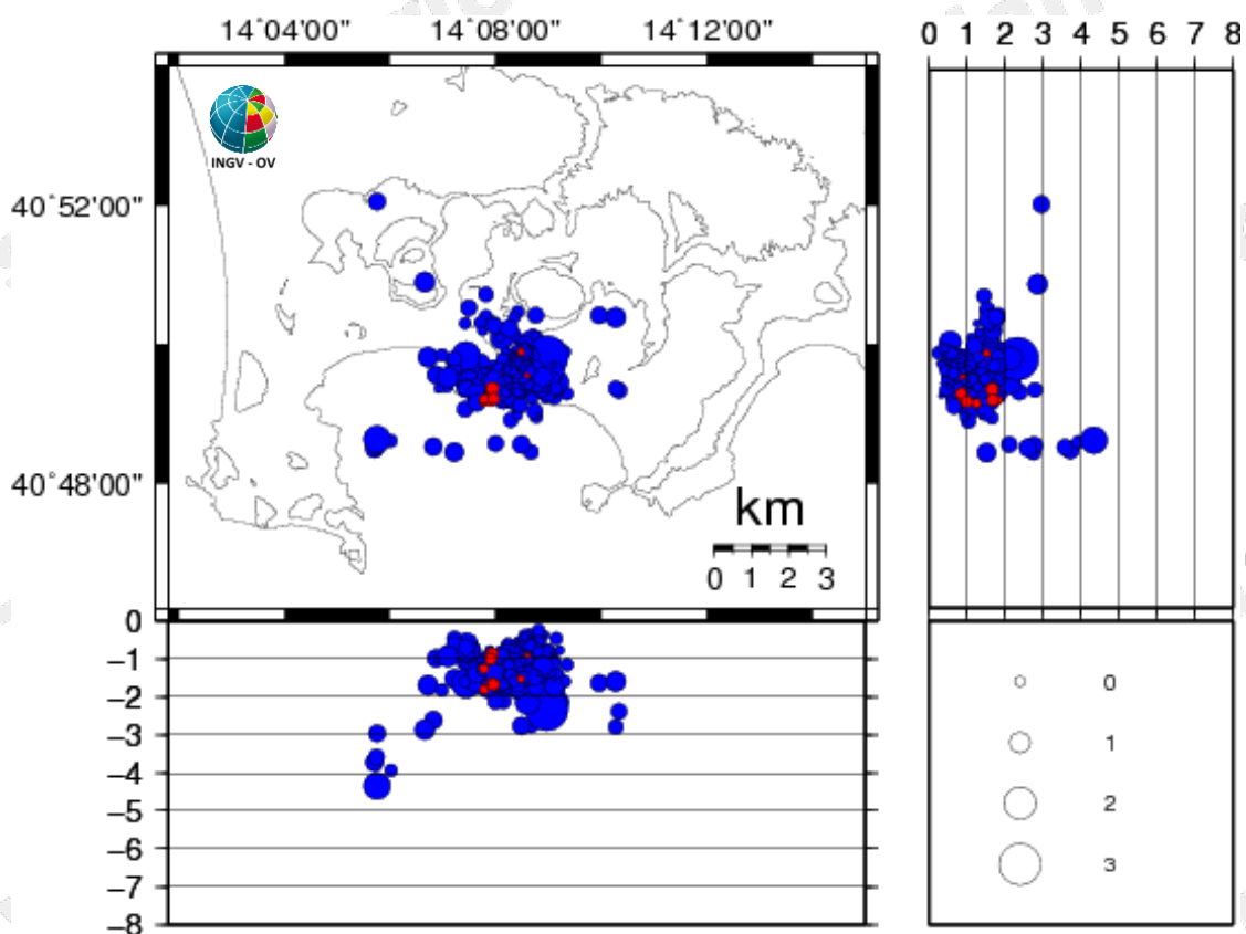
Figura 3.1 - Ipocentri dei terremoti localizzati ai Campi Flegrei negli ultimi 12 mesi (in totale 550). In rosso gli eventi localizzati nell'ultima settimana (in totale 9).
