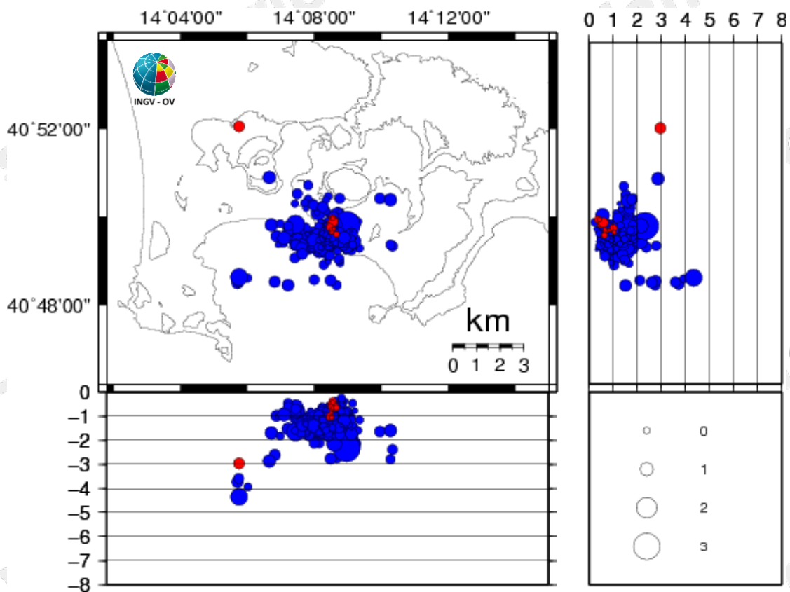
Figura 3.1 - Ipocentri dei terremoti localizzati ai Campi Flegrei negli ultimi 12 mesi (in totale 541). In rosso gli eventi localizzati nell'ultima settimana (in totale 11).
