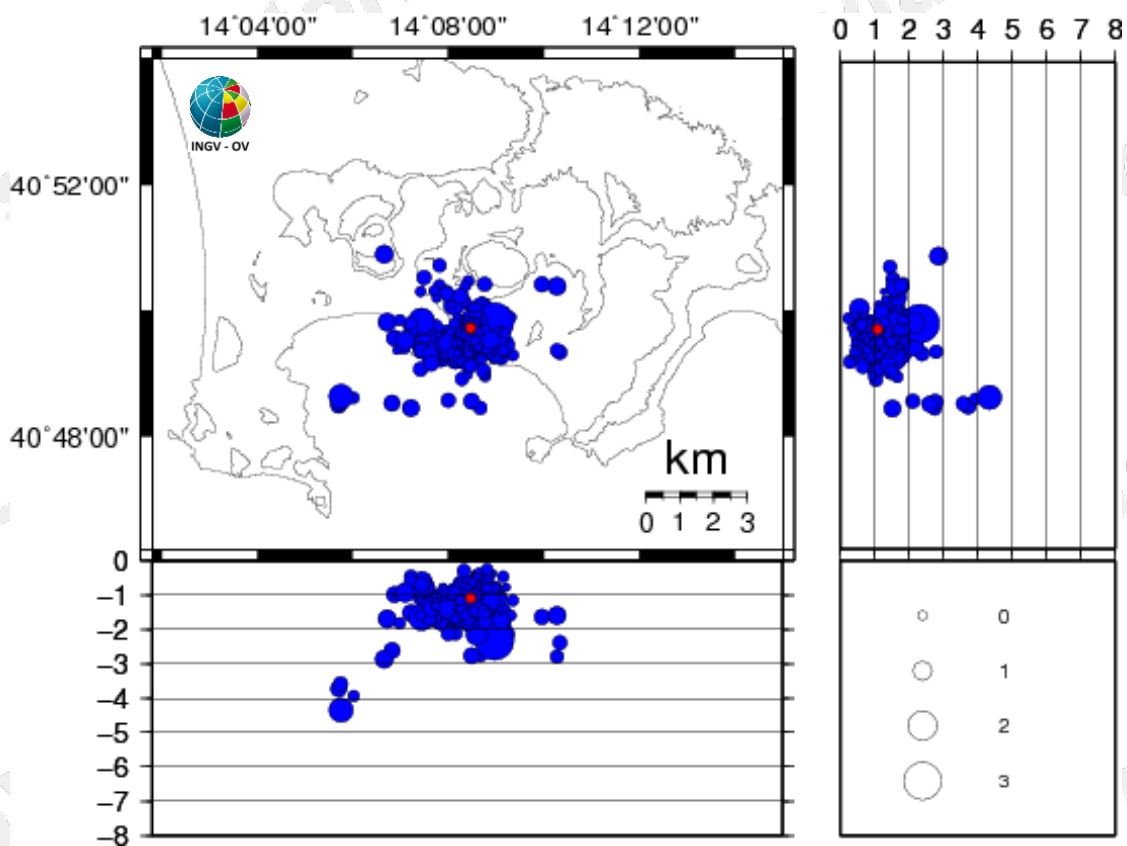
Figura 3.1 - Ipocentri dei terremoti localizzati ai Campi Flegrei negli ultimi 12 mesi (in totale 554). In rosso gli eventi localizzati nell'ultima settimana (in totale 1).
