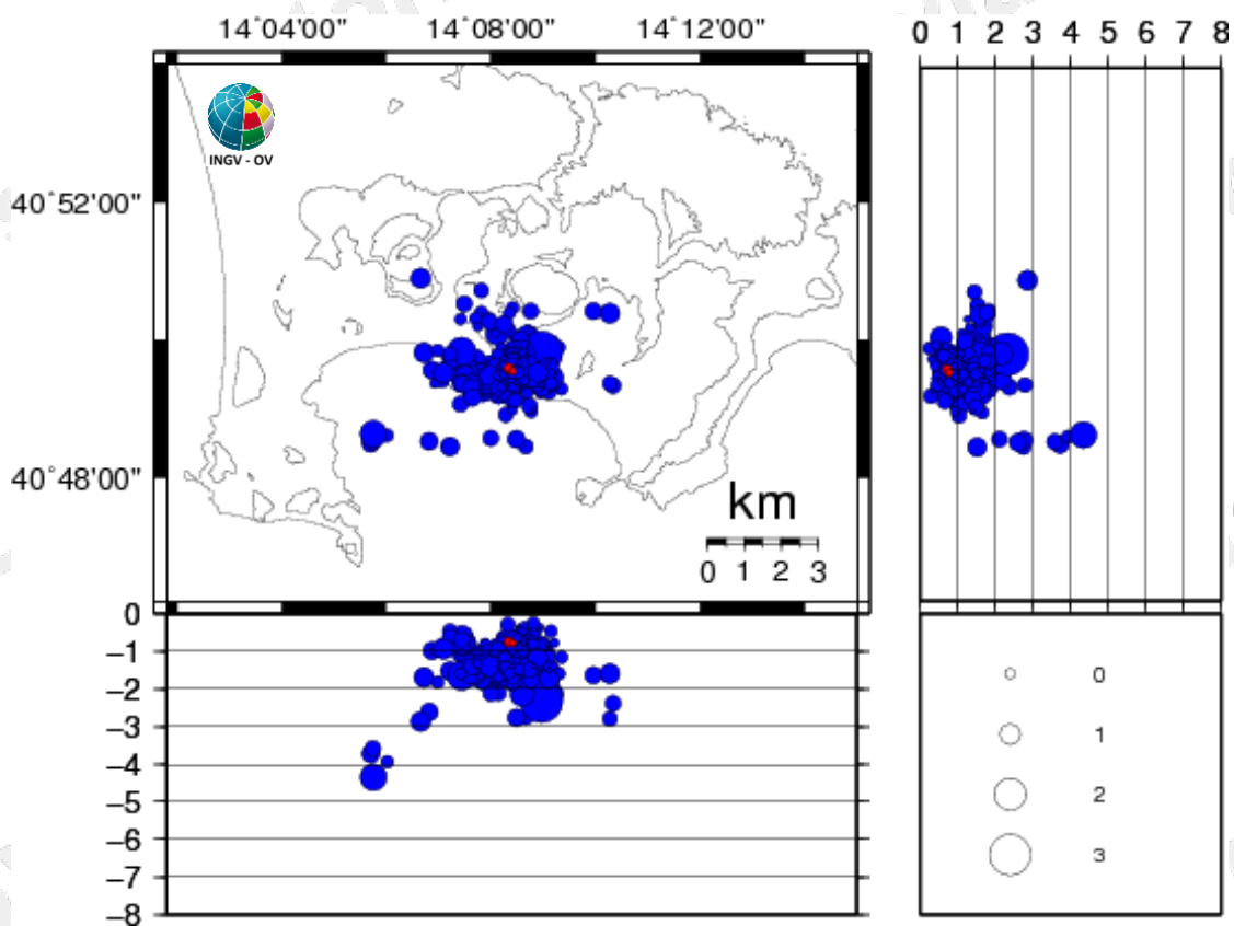
Figura 3.1 - Ipocentri dei terremoti localizzati ai Campi Flegrei negli ultimi 12 mesi (in totale 553). In rosso gli eventi localizzati nell'ultima settimana (in totale 2).
