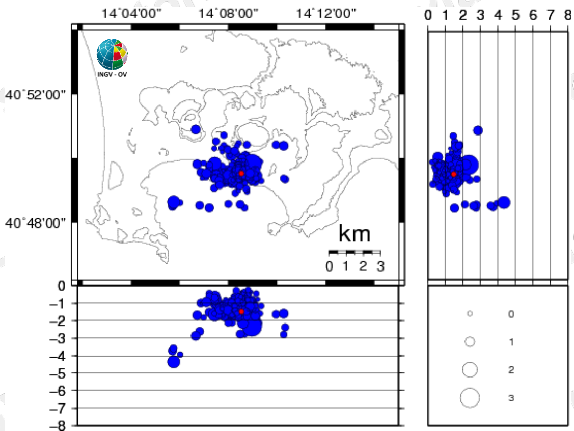
Figura 3.1 - Ipocentri dei terremoti localizzati ai Campi Flegrei negli ultimi 12 mesi (in totale 551). In rosso gli eventi localizzati nell'ultima settimana (in totale 1).
