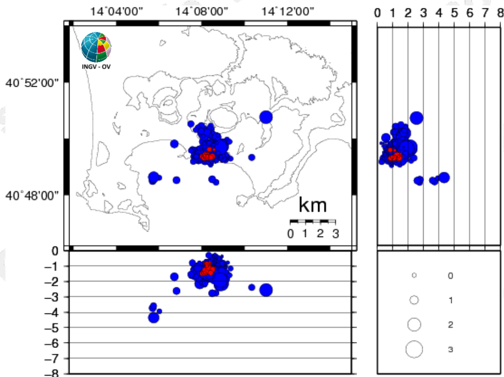
Figura 3.1 - Ipocentri dei terremoti localizzati ai Campi Flegrei negli ultimi 12 mesi (in totale 472). In rosso gli eventi localizzati nell'ultima settimana (in totale 16).
