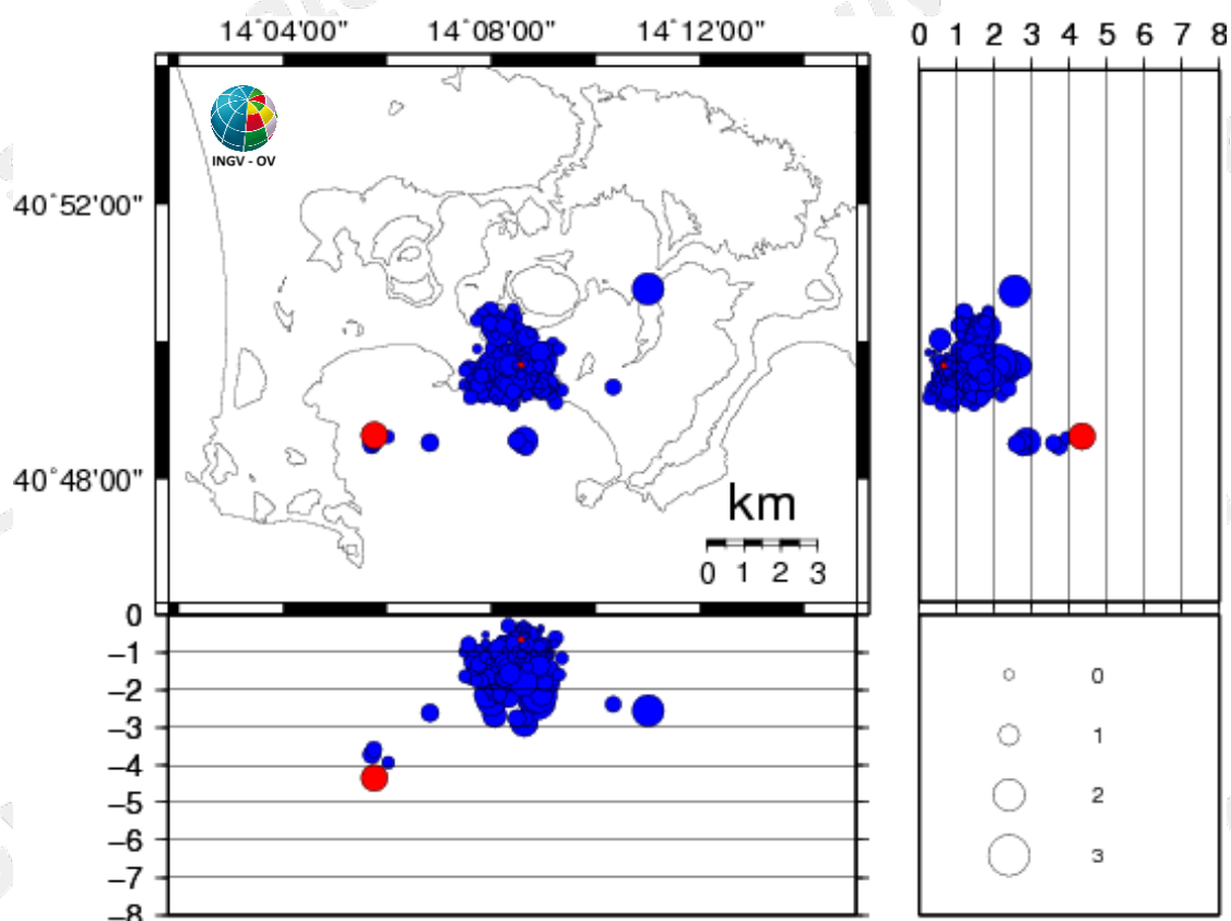
Figura 3.1 - Ipocentri dei terremoti localizzati ai Campi Flegrei negli ultimi 12 mesi (in totale 437). In rosso gli eventi localizzati nell'ultima settimana (in totale 2).
