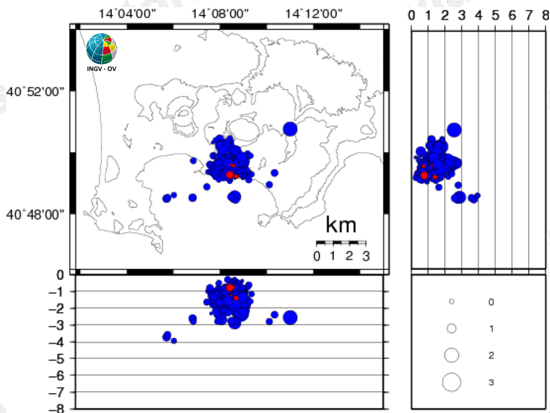
Figura 3.1 - Ipocentri dei terremoti localizzati ai Campi Flegrei negli ultimi 12 mesi (in totale 450). In rosso gli eventi localizzati nell'ultima settimana (in totale 4).
