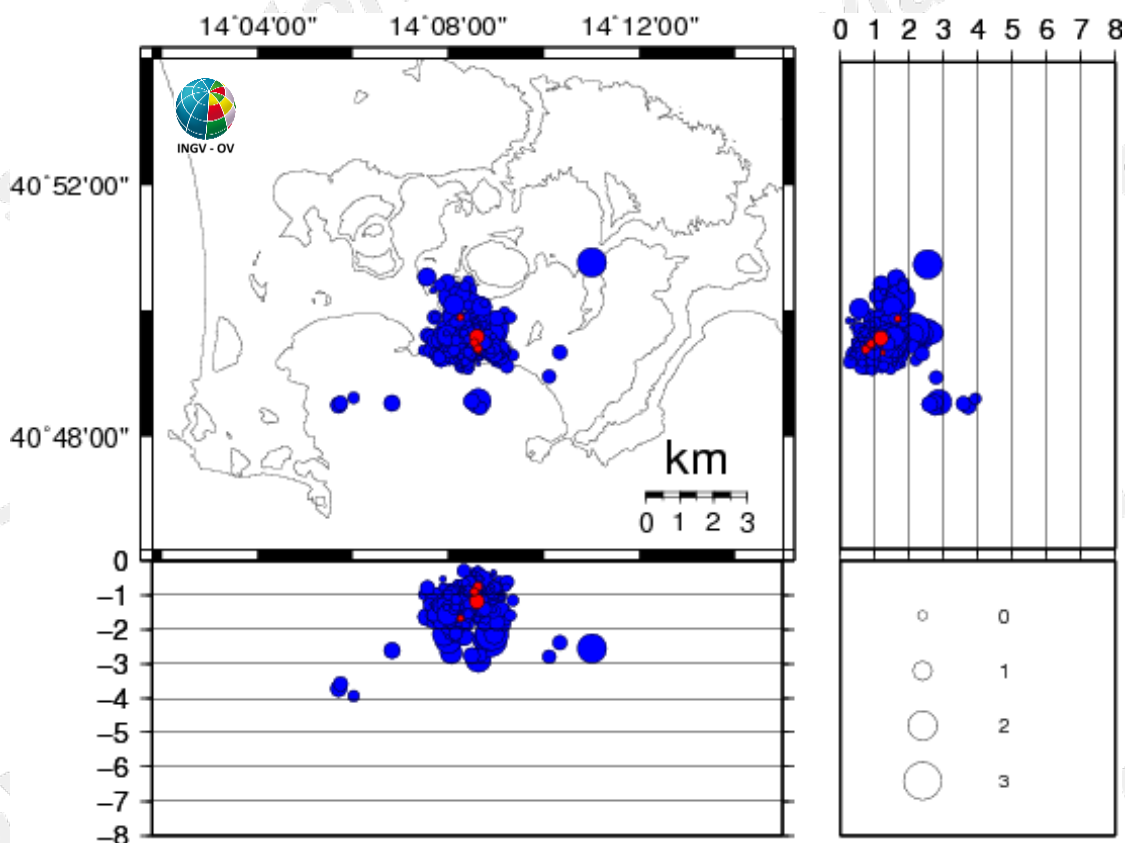
Figura 3.1 - Ipocentri dei terremoti localizzati ai Campi Flegrei negli ultimi 12 mesi (in totale 420). In rosso gli eventi localizzati nell'ultima settimana (in totale 5).
