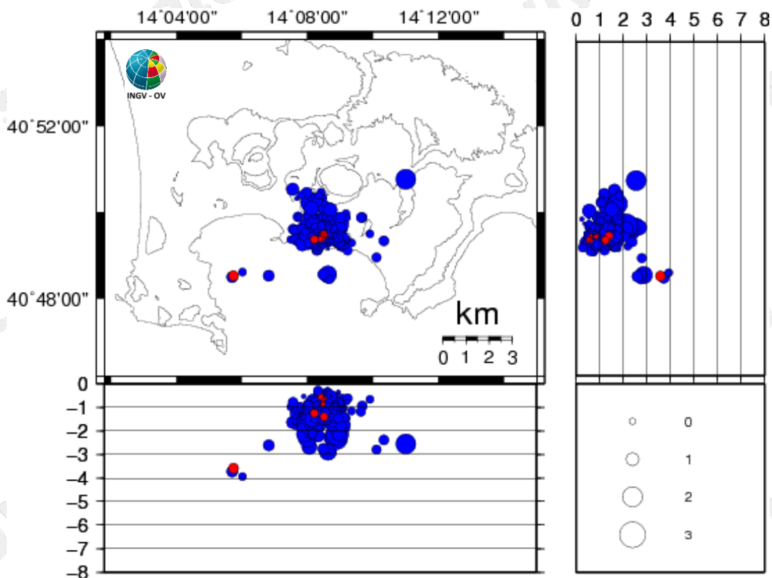
Figura 3.1 - Ipocentri dei terremoti localizzati ai Campi Flegrei negli ultimi 12 mesi (in totale 370). In rosso gli eventi localizzati nell'ultima settimana (in totale 7).
