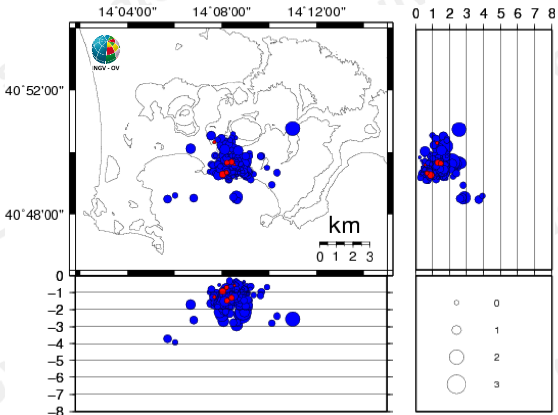
Figura 3.1 - Ipocentri dei terremoti localizzati ai Campi Flegrei negli ultimi 12 mesi (in totale 369). In rosso gli eventi localizzati nell'ultima settimana (in totale 7).
