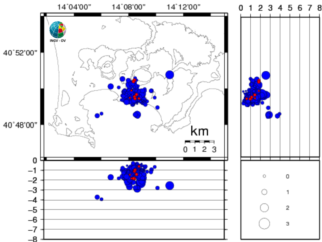
Figura 3.1 - Ipocentri dei terremoti localizzati ai Campi Flegrei negli ultimi 12 mesi (in totale 322). In rosso gli eventi localizzati nell'ultima settimana (in totale 9).
