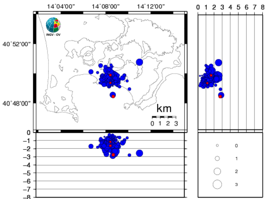
Figura 3.1 - Ipocentri dei terremoti localizzati ai Campi Flegrei negli ultimi 12 mesi (in totale 279). In rosso gli eventi localizzati nell'ultima settimana (in totale 3).
