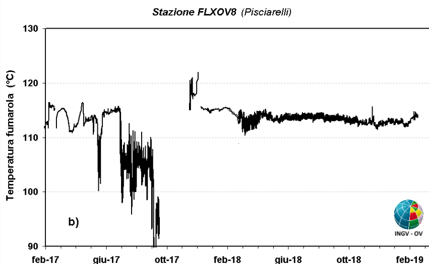
Figura 5.1 - (a) Valori del flusso di CO 2 dal suolo (medie giornaliere); (b) dettaglio della temperatura della fumarola dal mese di febbraio 2017.
