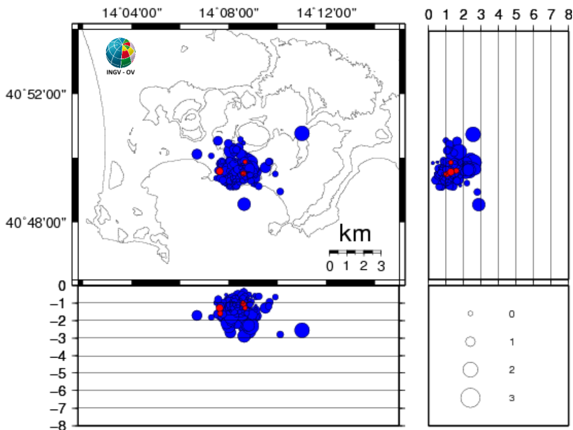
Figura 3.1 - Ipocentri dei terremoti localizzati ai Campi Flegrei negli ultimi 12 mesi (in totale 280). In rosso gli eventi localizzati nell'ultima settimana (in totale 5).
