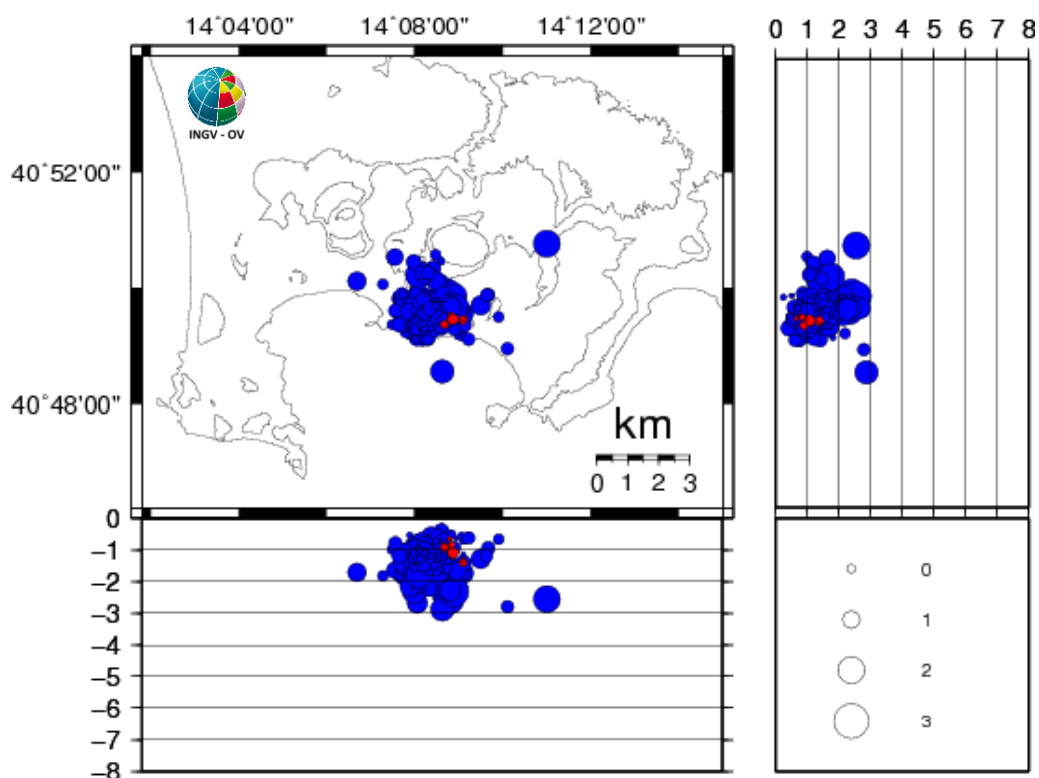
Figura 3.1 - Ipocentri dei terremoti localizzati ai Campi Flegrei negli ultimi 12 mesi (in totale 389). In rosso gli eventi localizzati nell'ultima settimana (in totale 6).
