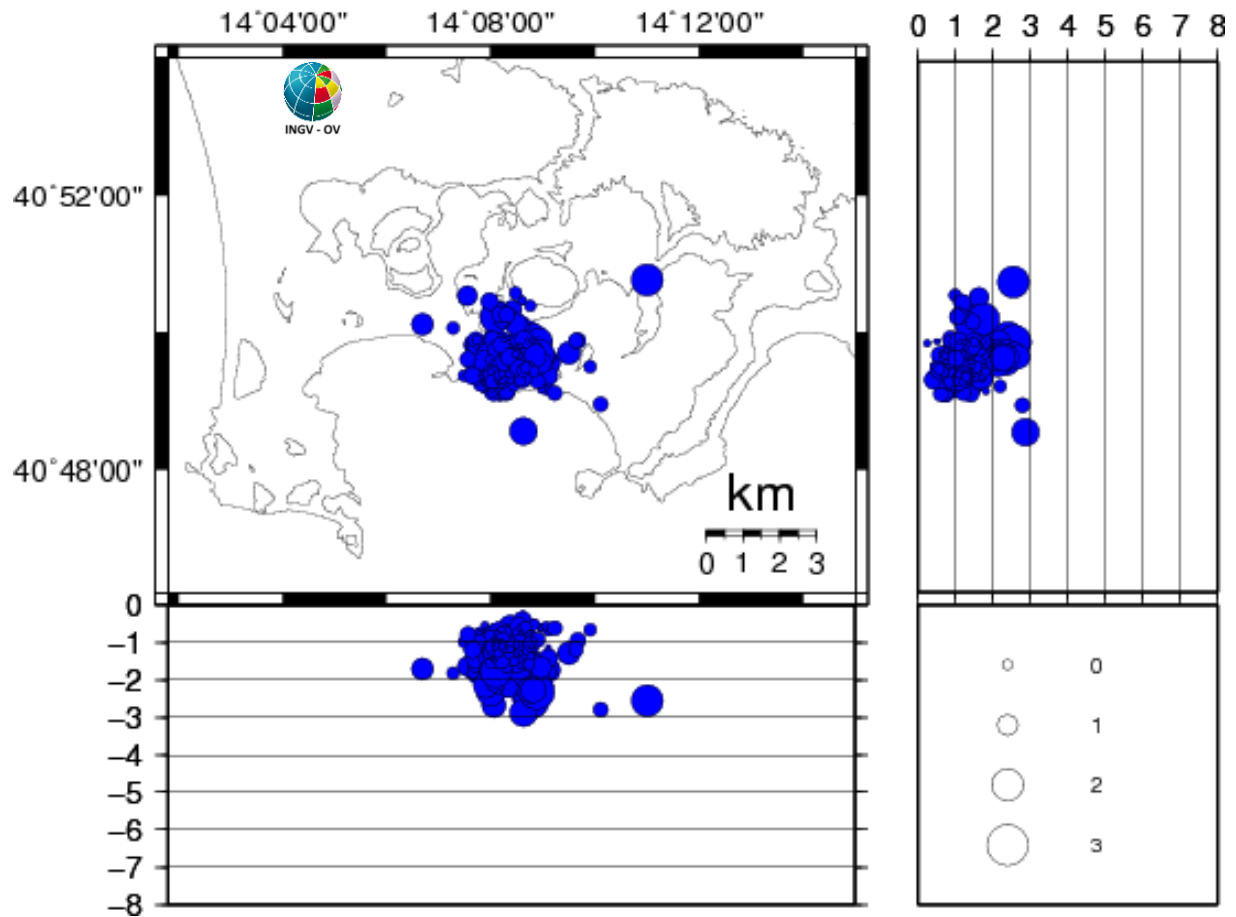
Figura 3.1 - Ipocentri dei terremoti localizzati ai Campi Flegrei negli ultimi 12 mesi (in totale 298).
