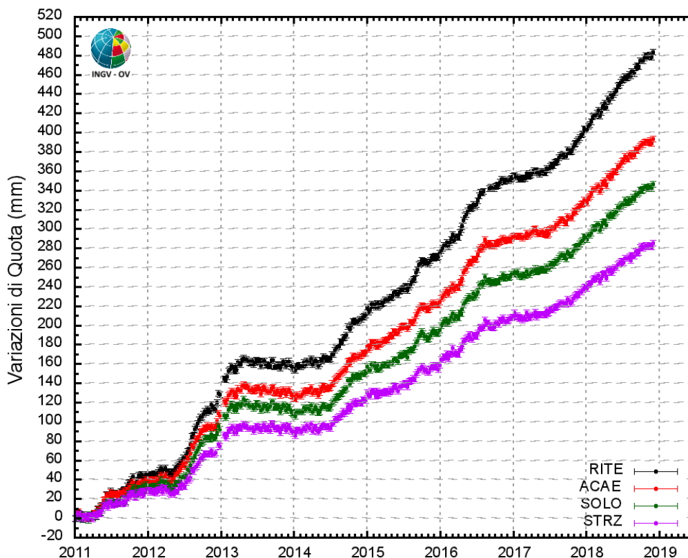
Figura 4.1 - Serie temporali delle variazioni in quota delle stazioni di RITE (Pozzuoli – Rione Terra), ACAE (Accademia Aeronautica), SOLO (Solfatarata) e STRZ (Pozzuoli - Cimitero) dal 01 gennaio 2011 al 01 dicembre 2018.
