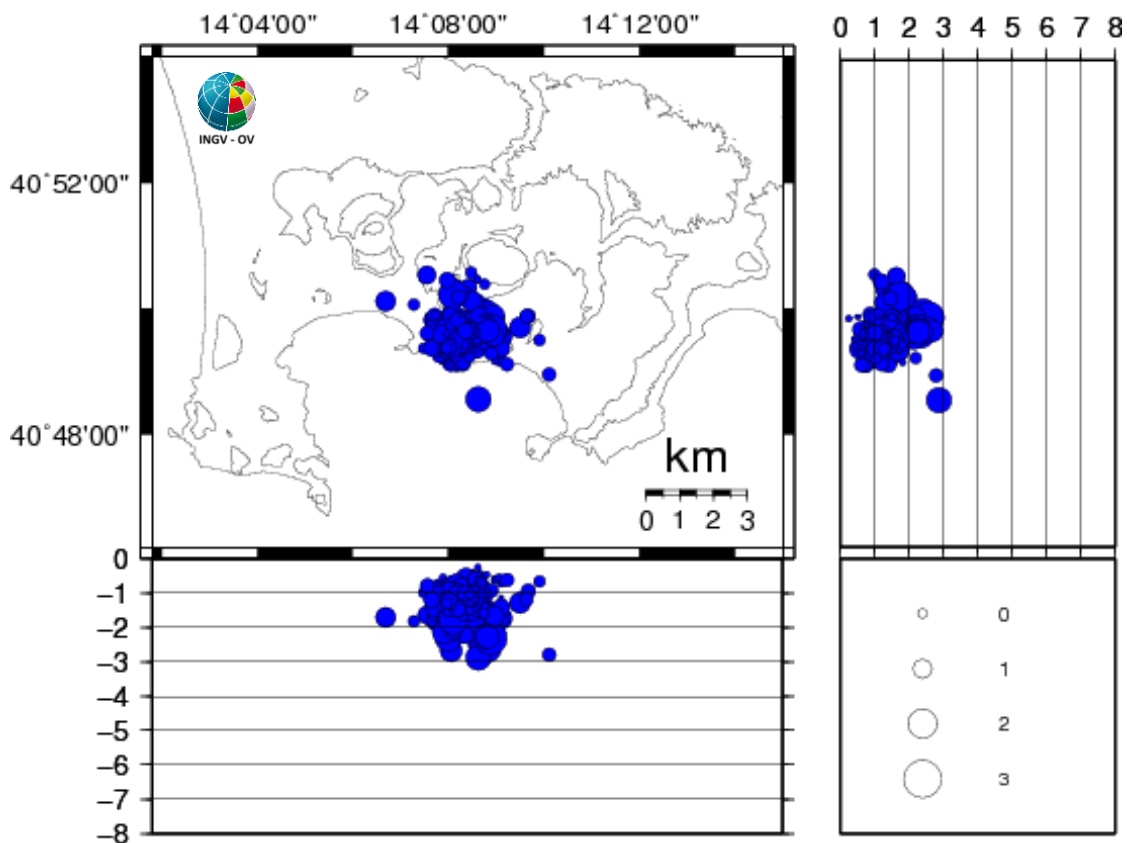
Figura 3.1 - Ipocentri dei terremoti localizzati ai Campi Flegrei negli ultimi 12 mesi (in totale 293).
